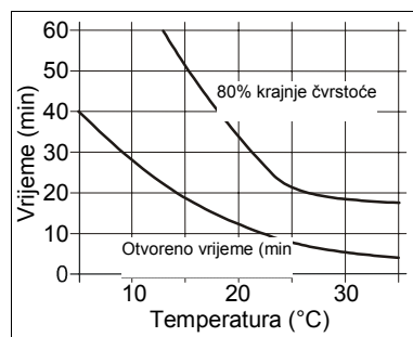
Dijagram: Otvoreno vrijeme i brzina otvrdnjavanja za SikaFast®-5221
