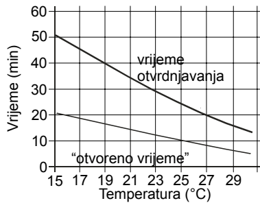
Dijagram 1: "otvoreno vrijeme" i vrijeme otvrdnjavanja za SikaForce®-7110 L25
